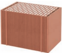
Füllung: Perlite-Dämmstoff \lambda = 0,09 \text{ W/mK} R_w^{(1)} \geq 50 \text{ dB} f_k = 5,3 \text{ MN/m}^2 (bei SFK 12)
