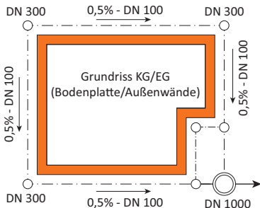
Beispiel Ringdränung (Mindestabmessungen) nach DIN 4095 Ziegellexikon Mauerwerk 2020 ISSN 2193-293X
