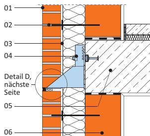
Winkelkonsolanker zur Lastabfangung von Verblendmauerwerk
