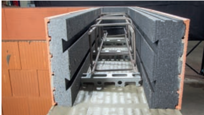
Ziegel-Wärmedämmschale mit bauseits eingebrachtem Bewehrungskorb auf Abstandhaltern vor dem Betoniervorgang..
