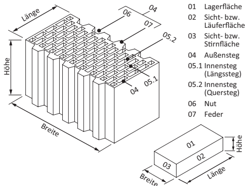
Allgemeine Bezeichnungen bei einem Hochlochziegel (Bild links) und einem Vollziegel (Bild rechts)
