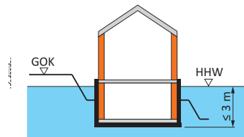
W2.1-E | Hohe Einwirkung von drückendem Wasser © Ziegel Zentrum Süd e. V. www.ziegel.com
