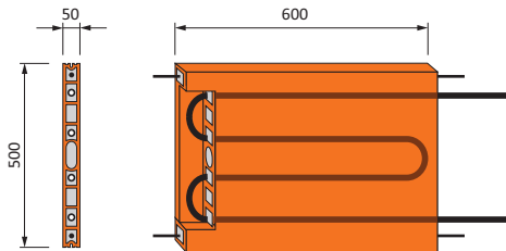
Ziegelheizelement: Langlochziegel mit integriertem Heizstrang
