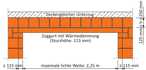
Geometrische Randbedingungen für Flachstürze mit 113 mm hohen Zugurten mit Wärmedämmung und einlagiger Übermauerung
