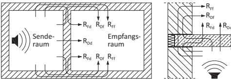
Schallübertragung über das trennende Bauteil ( R_{Dd,w} ) und die flankierenden Bauteile ( R_{Ff} , R_{Fd} , R_{Df} ) horizontal und vertikal
