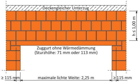
Geometrische Randbedingungen für Flachstürze mit 71 oder 113 mm hohen Zugurten ohne Wärmedämmung und mehrlagiger Übermauerung
