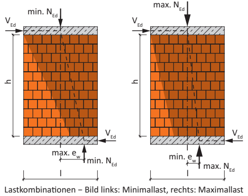
Lastkombinationen – Bild links: Minimallast, rechts: Maximallast
